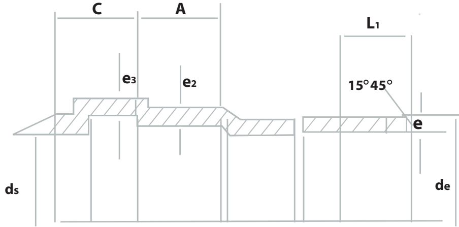
Şekil 1: Boru Başı ve Boru Ucu Boyutları
